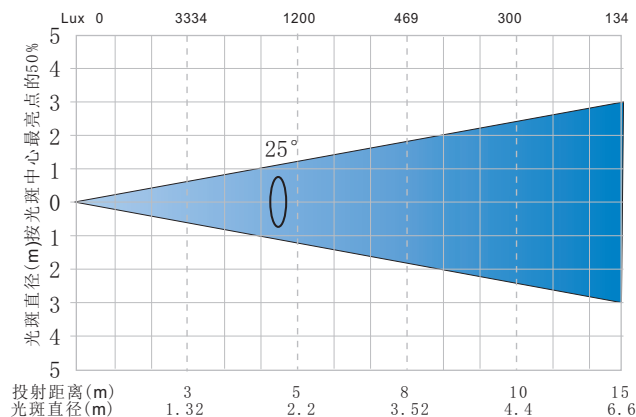
高显 (CRI) 灯珠 LP-1915 4*1 RGBW
