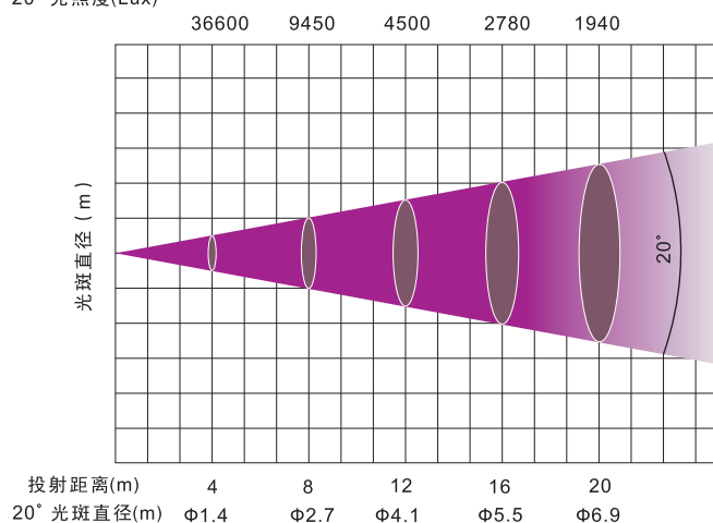
20° 光照度(Lux)
